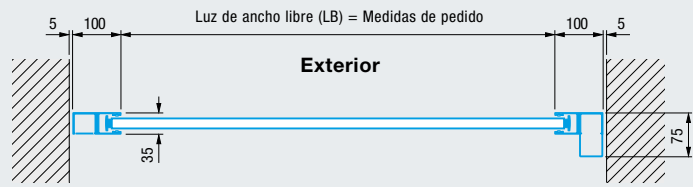
Montaje en el hueco
