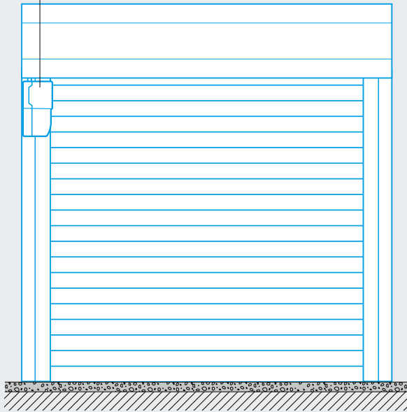
Automatismo (cadena de tracción manual) interior izquierda
