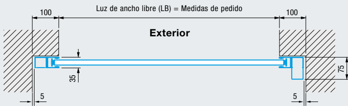
Montaje detrás del hueco
