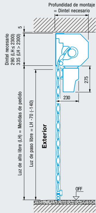
Montaje en el hueco
